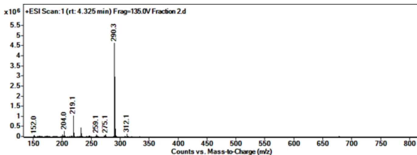
Figure S 5. LCMS (+) ESI data of mesembrine
